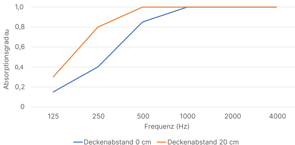
HOFA Deckensegel, Materialstärke: 4 cm Messung der Schallabsorption im Hallraum
