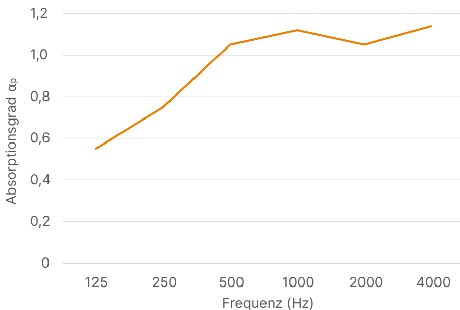
HOFA Tischtrennwand, Materialstärke: 4 cm Messung der Schallabsorption im Hallraum
